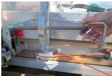
Frästiefe einstellen: mit Niro-Spindel und Markierung.
